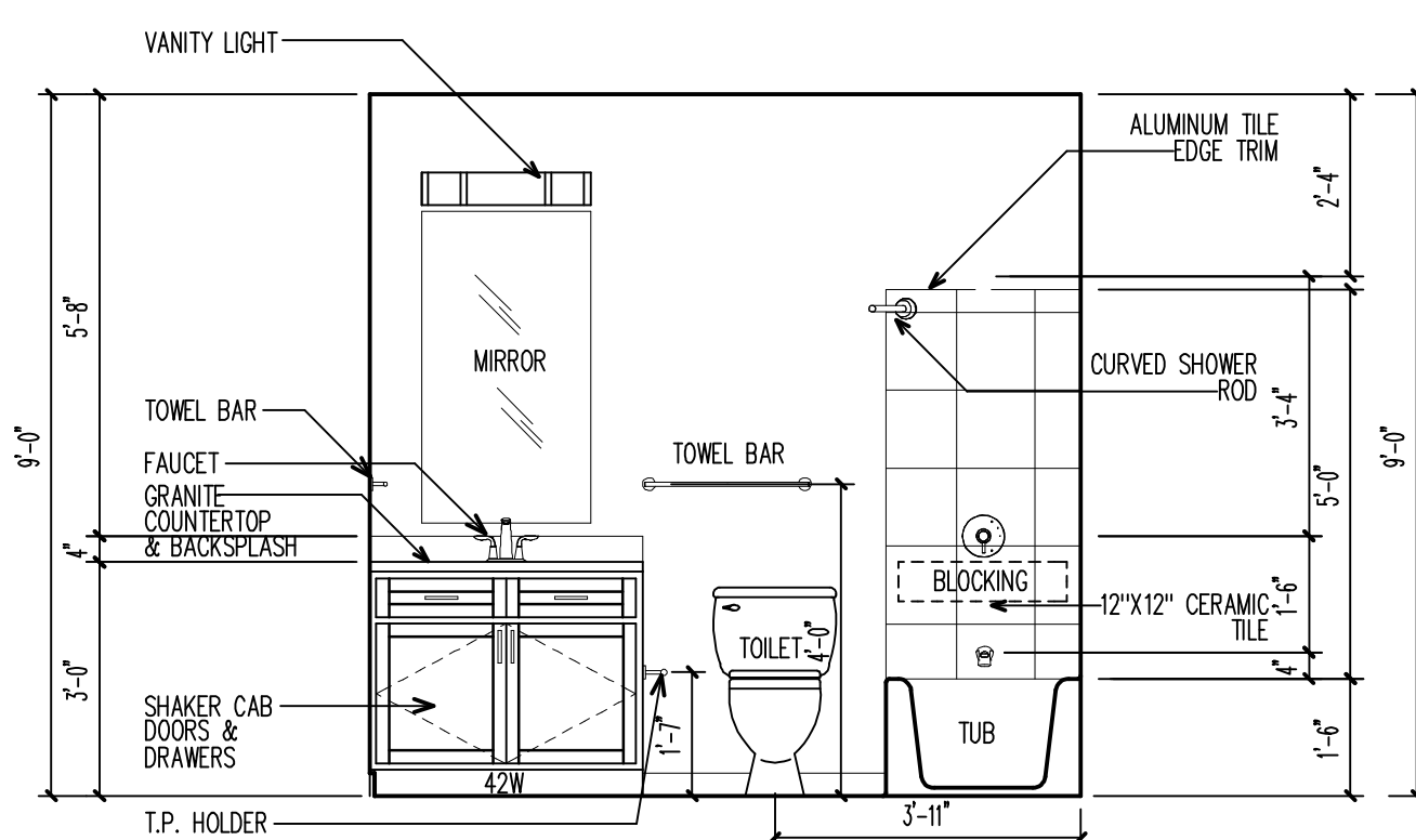
05 BATH ELEVATION SCALE: 3/8" = 1'-0"
