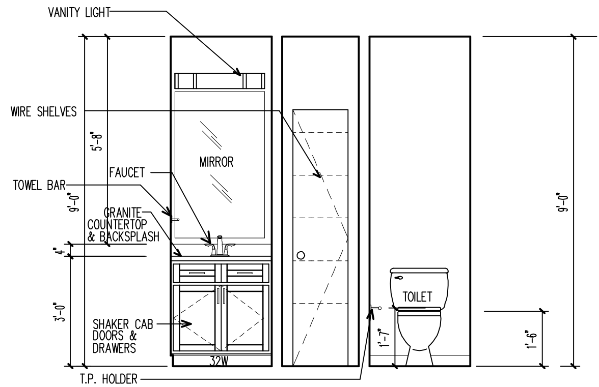
05 BATH ELEV. (TYP.) SCALE: 3/8" = 1'-0"
