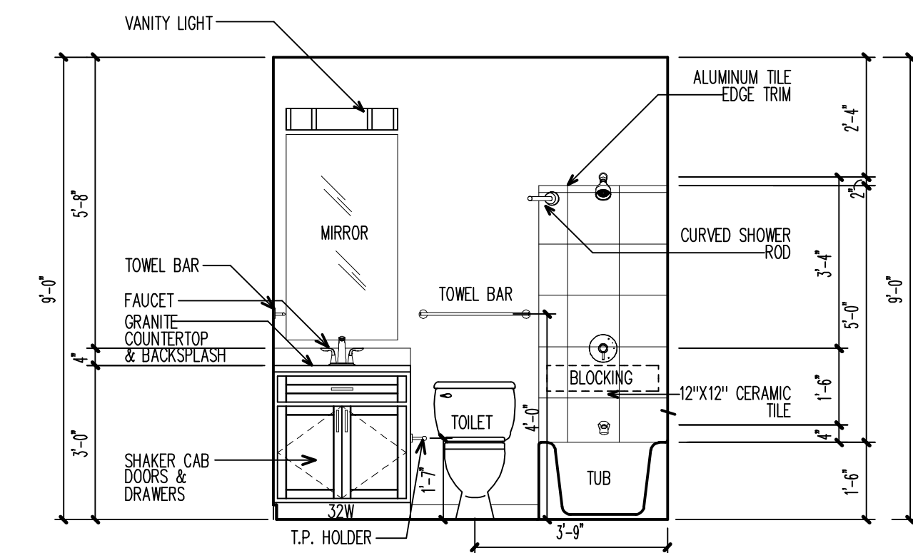
05 BATHS (TYP.) SCALE: 3/8" = 1'-0"
